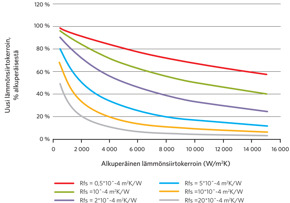
Kuva 2 Putkivirtauksen sisäpuolisen likavastuksen ( R_{f,s} ) vaikutus kokonaislämmönsiirtokerroimeen (Pöyry).
